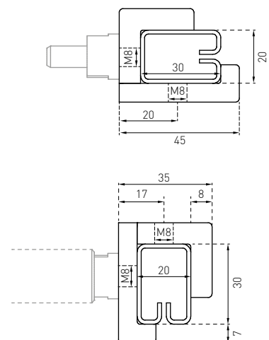
CX3-P-H90: zweifach positionierbar_dual use
